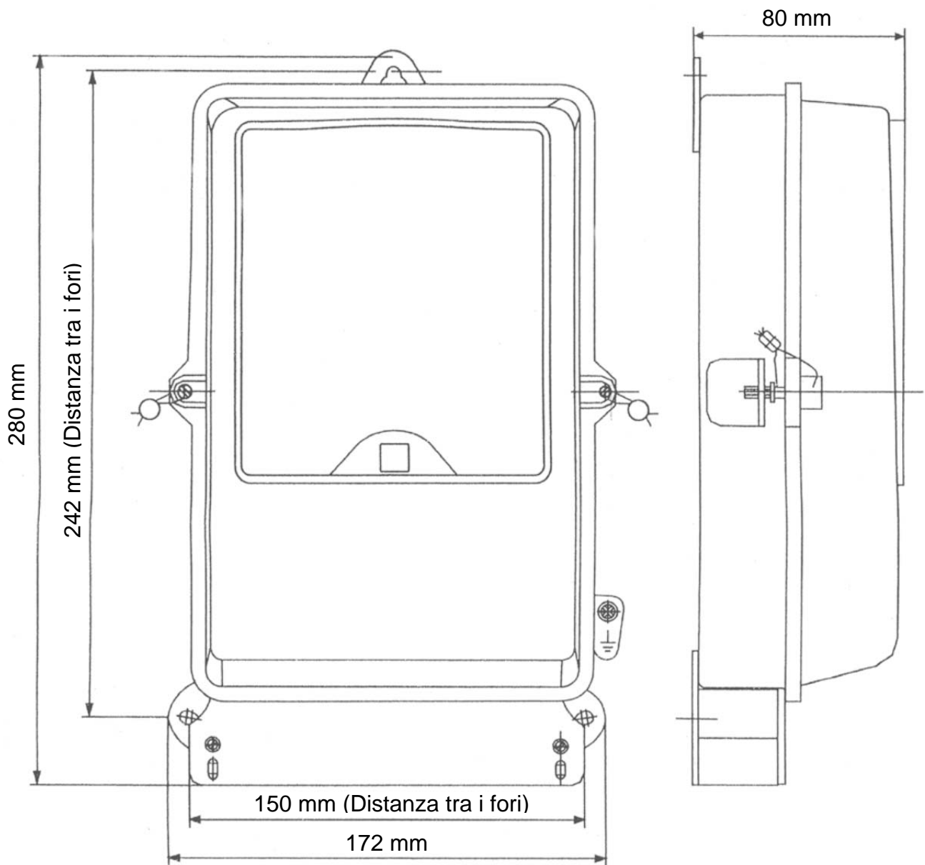
Dimensioni del DTS e distanza tra le viti di fissaggio.
